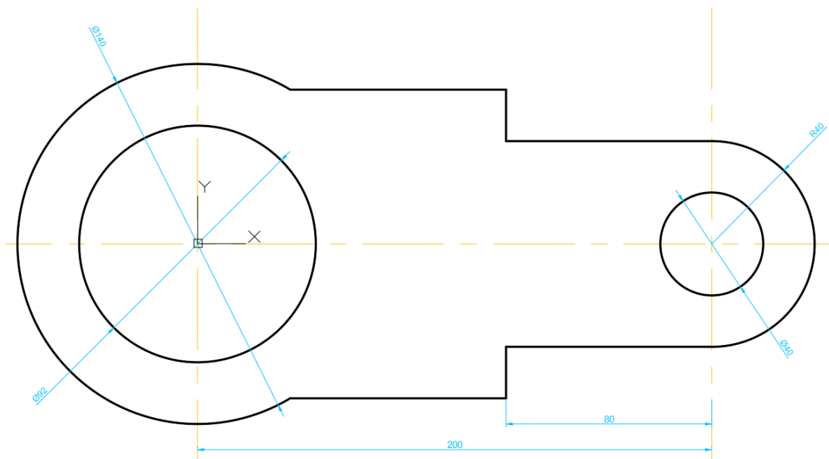
Рисунок 1.7 – Початкові розміри
