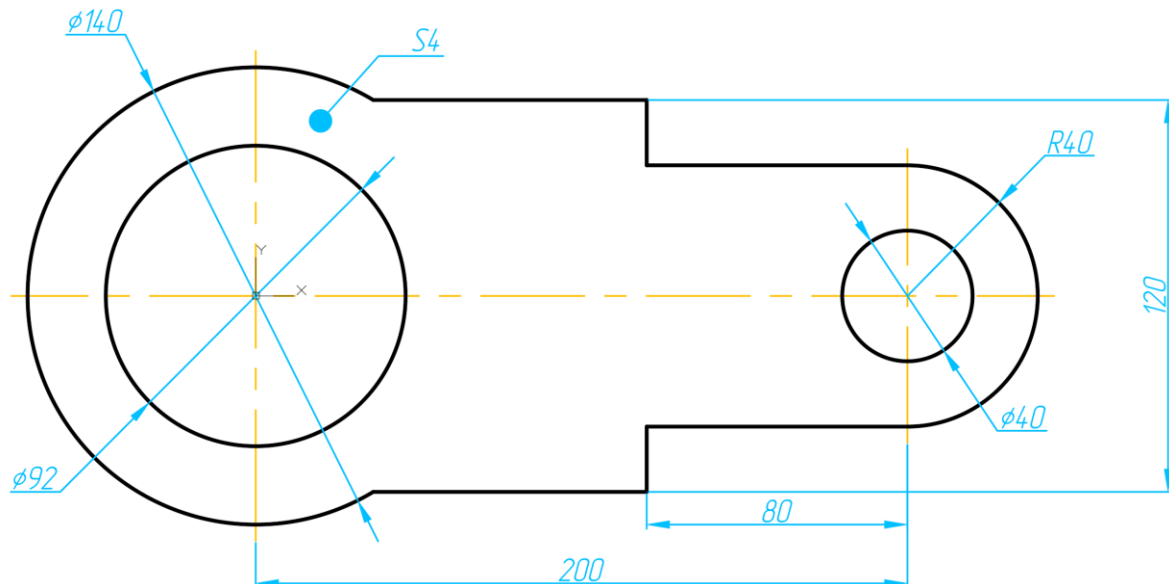
Рисунок 1.15 – Завершений кресленник
